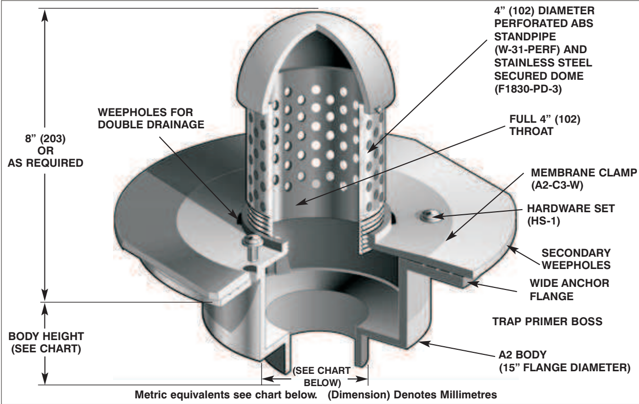
A2 Body
