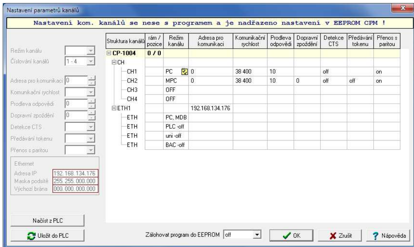
Obr.7.1 Nastavení parametrů centrální jednotky
