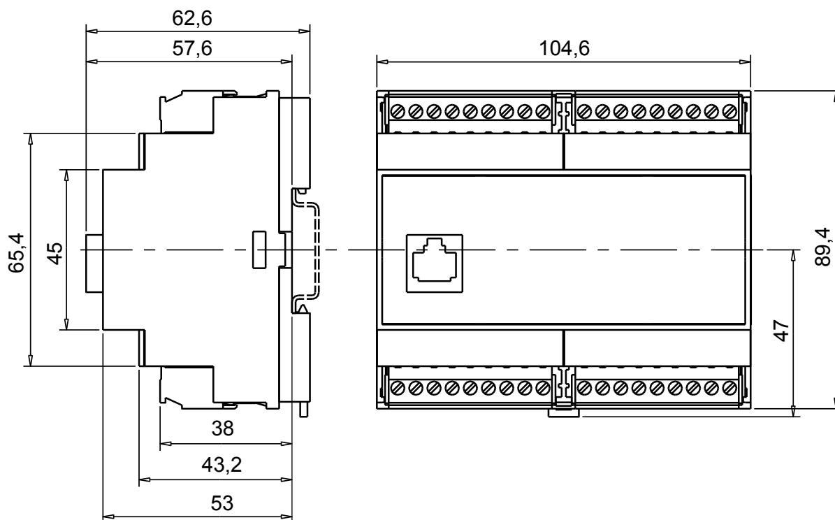
Obr.2.2 Rozměry základních modulů CP-10x4 v provedení s vyjímatelnými svorkovnicemi
