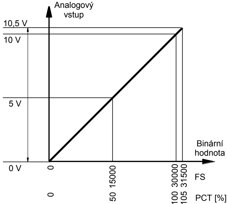
Obr.4.12 Napěťový rozsah analogových vstupů modulů CP-10x4
