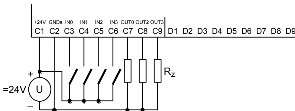
Obr.3.3 Typický příklad připojení spínačů a zátěží k základnímu modulu při osazeném submodulu PX-7812 na kanálu CH2
