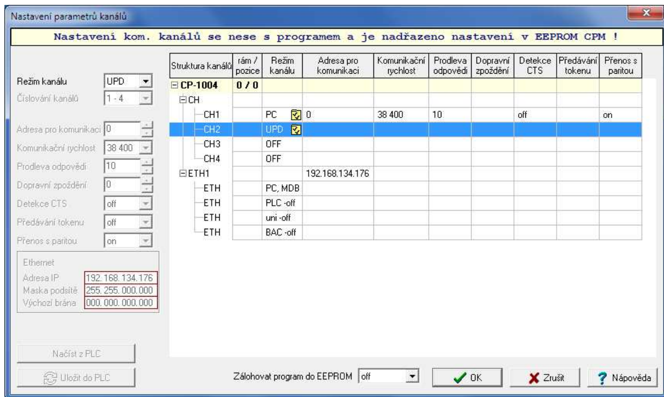
Obr.3.4 Výběr režimu UPD na kanálu CH2
