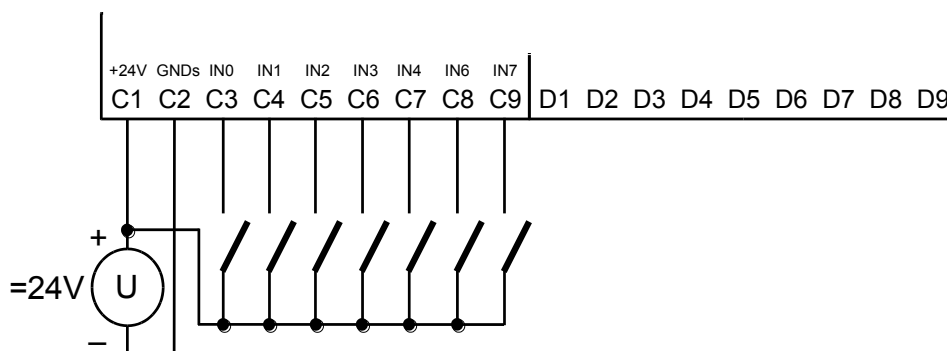
Obr.3.2 Typický příklad připojení spínačů k základnímu modulu při osazeném submodulu PX-7811 na kanálu CH2
