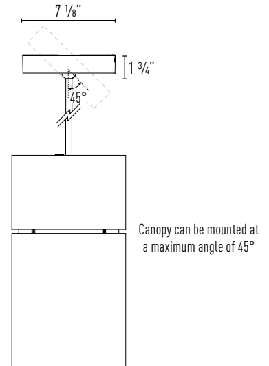
Pendant Mount
