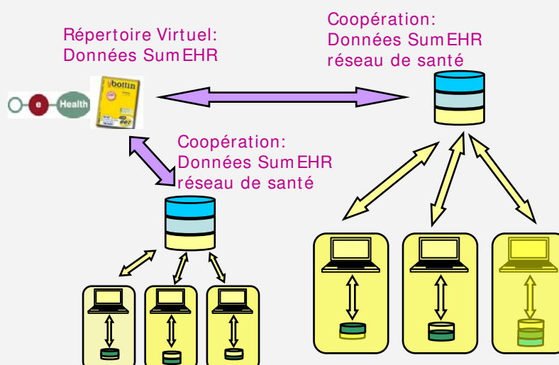
Figure 12 : SumEHR: Proposition d'Architecture pour les données médicales
