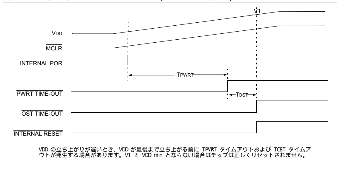
図 8-13：電源 CN 時のタイムアウトシーケンス（MCLR は VDD に接続）：VDD の立ち上がりが遅い
