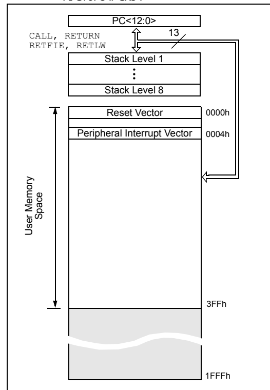
図 4-2: プログラムメモリとスタック配置図 - PIC16F84/CR84
