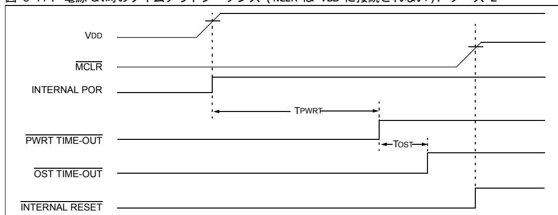
図 8-11：電源 ON 時のタイムアウトシーケンス ( \overline{\text{MCLR}} は VDD に接続されない)：ケース 2
