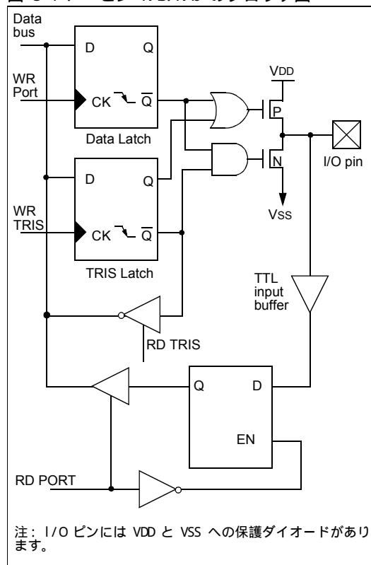
図 5-1 : ピン RA3: RA0 のブロック図
