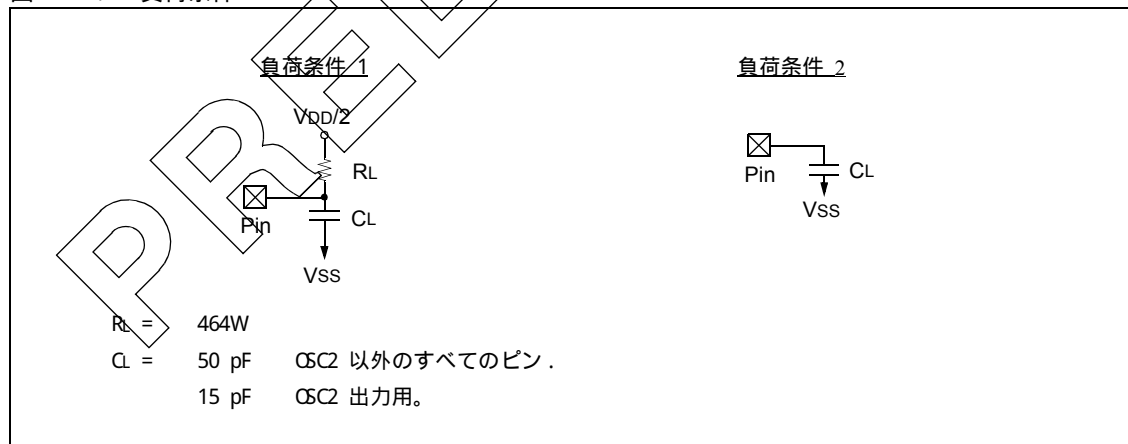
図 11-2: 負荷条件
