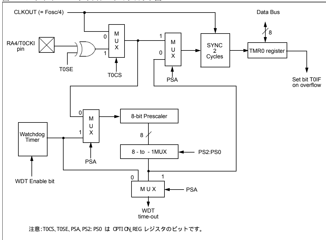
図 6-6: タイマ / WDT プリスケアラのブロック図
