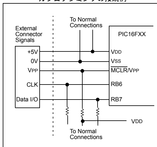
図 8-20 標準的なインターサーキットシリアルプログラミングの接続例
