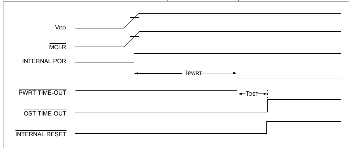
図 8-13：電源 CN 時のタイムアウトシーケンス（MCLR は VDD に接続）：VDD の立ち上がりが遅い
