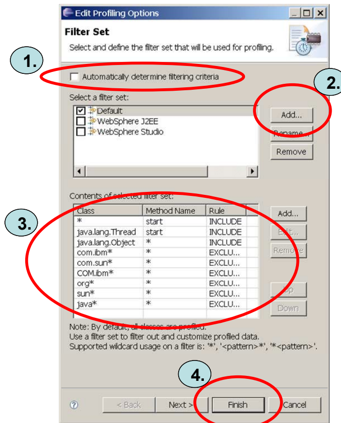
Figure 12. Edit profiling options dialog.
