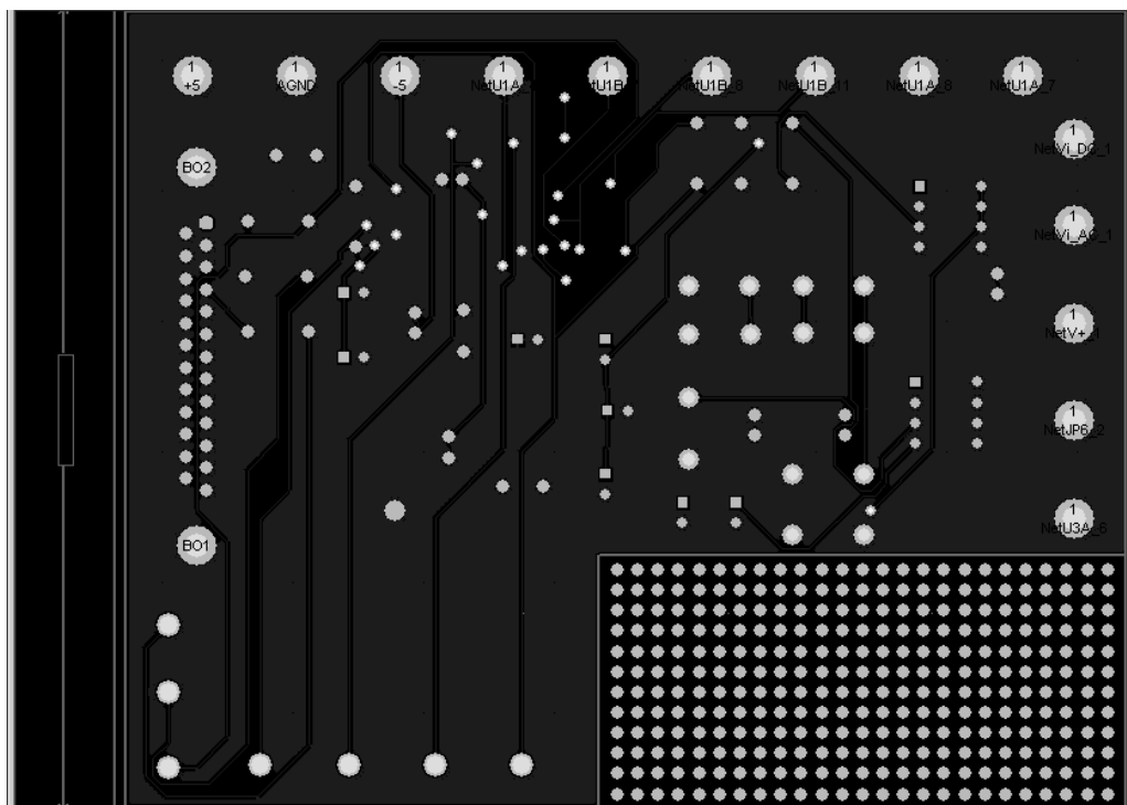
Figure 19. Bottom Layer
