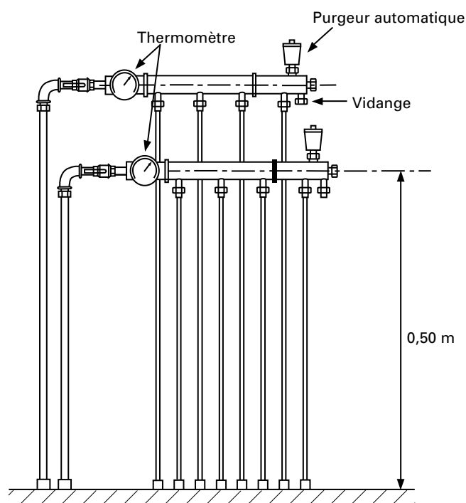
▲ Figure 27 : Fixation des collecteurs à 0,50 m du sol
