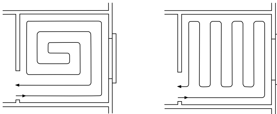
▲ Figure 32 : Les deux méthodes de pose d'un plancher chauffant : en spirale et en serpentin
