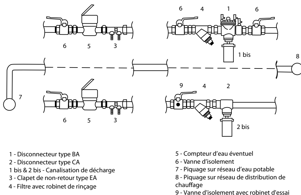
▲ Figure 15 : Constitution de l'ensemble du dispositif de protection
