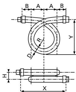
Raccordement en cor de chasse
