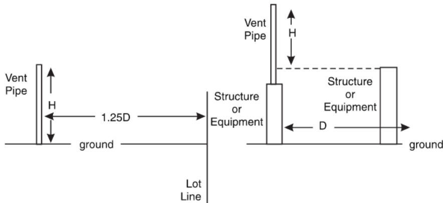
FIGURE 2209.5.4.3.4 HYDROGEN VENT PIPE HEIGHT (H) VERSUS DISTANCE (D) REQUIREMENTS
