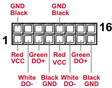
USB2 Header
