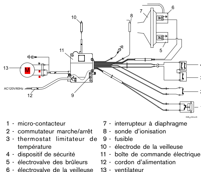
Fig. 14 - Schéma des circuits électriques
