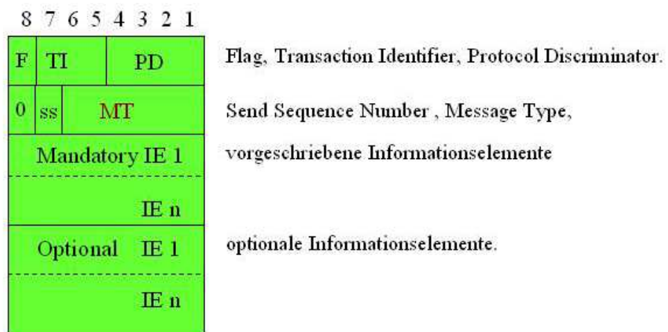
Bild 29: Aufbau eines Rahmens der Schicht 3
