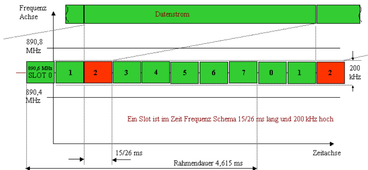
Bild 16: Zeiteilung der zur Verfügung stehenden Frequenzen
