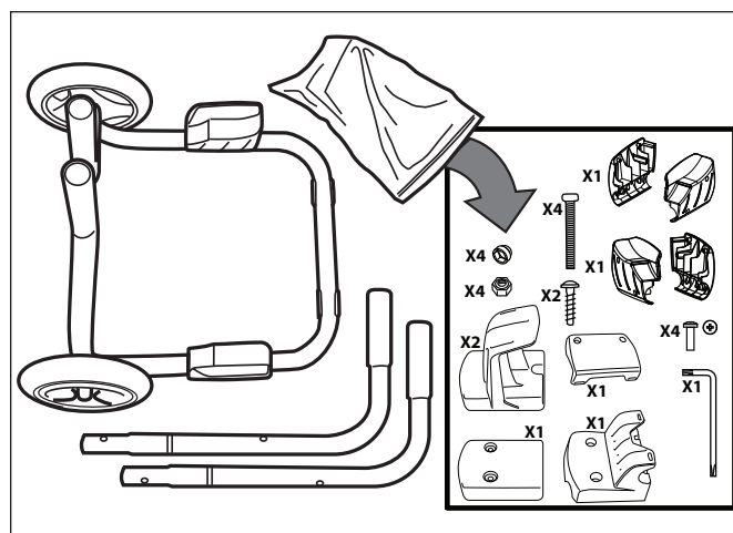
Figura 1. Componentes del Limpiafondos
