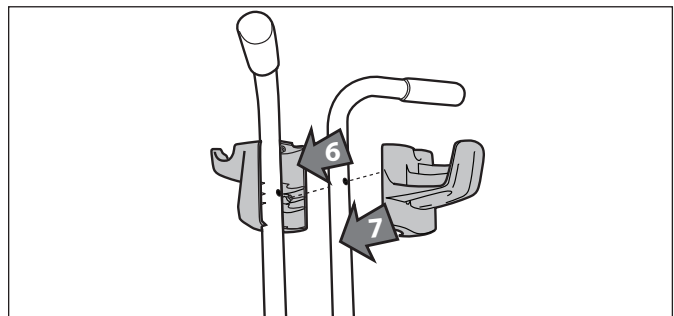
Figura 6. Instale los soportes en las manijas superiores
