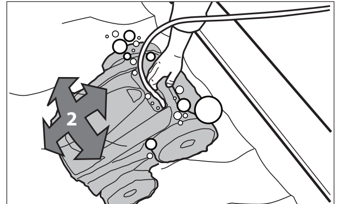
Figure 17. Nettoyeur au fond de la piscine
