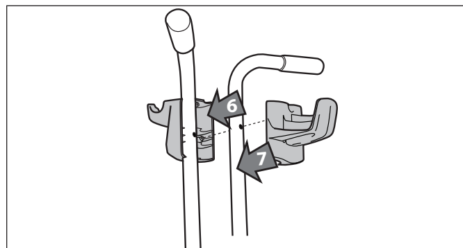
Figure 6. Installer les crochets sur les poignées supérieures
