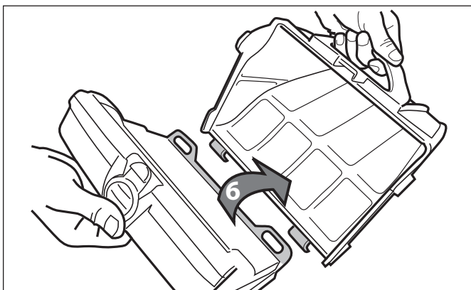
Figura 27. Remueva el porta Filtro
