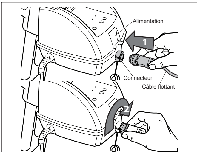
Figure 15. Raccordement électrique
