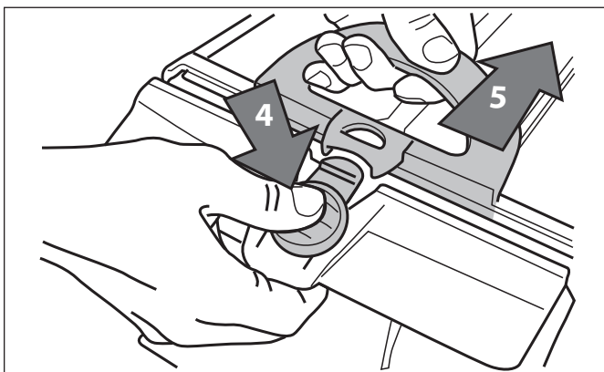
Figura 26. Abra el ensamble del filtro
