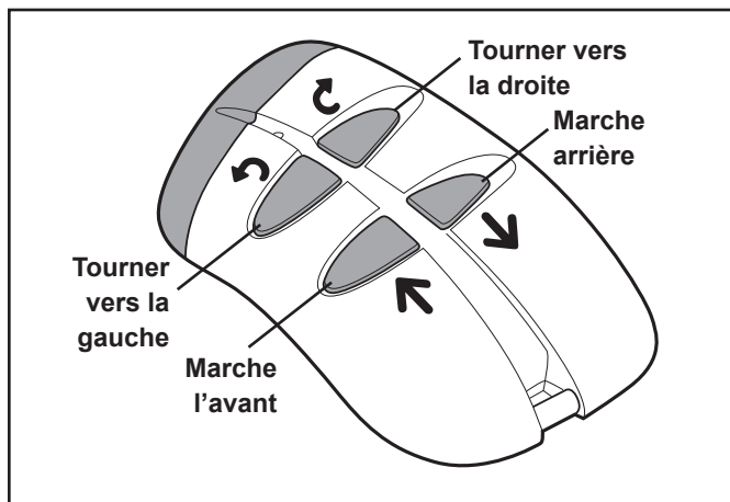
Figure 23. Télécommande
