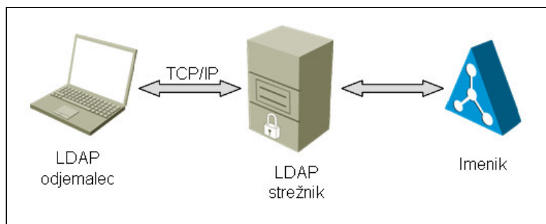
Slika 2.3: LDAP strežnik
