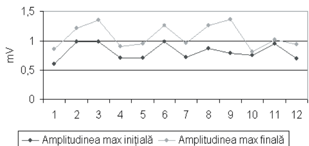
Fig. 5 – Valorile maxime ale amplitudinii semnalului EMG în CVM efectuate înainte și după CV 70% până la epuizare, la sportivi antrenati în regim de rezistență.
