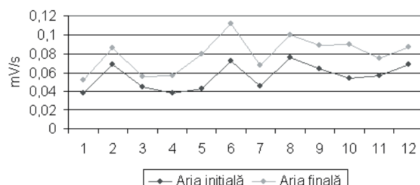
Fig. 7 – Aria semnalului EMG în CVM efectuate înainte și după CV 70% până la epuizare, la sportivi antrenati în regim de rezistență.
