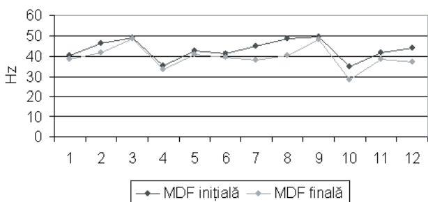
Fig. 6 – Valorile frecvențelor mediane ale semnalului EMG în CVM efectuate înainte și după CV 70% până la epuizare, la lotul de sportivi antrenati în regim de rezistență.
